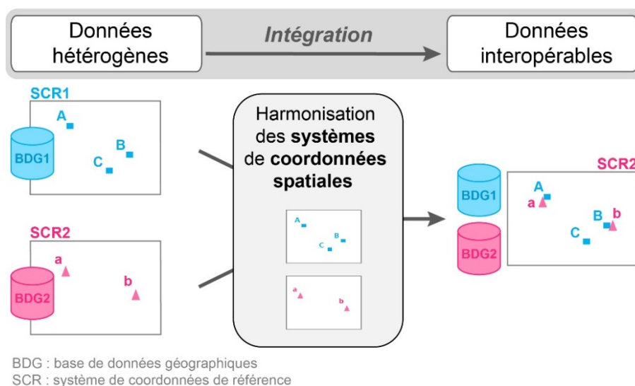
Figure 2.5. Intégration minimale pour la superposition visuelle : harmonisation des systèmes de coordonnées spatiales
